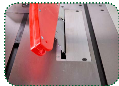
Pilový kotouč je sklopný vlevo v úhlu 0° až -45°
